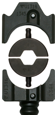
Outer die holder V1318, BNP dies, inner die holder V1316.
